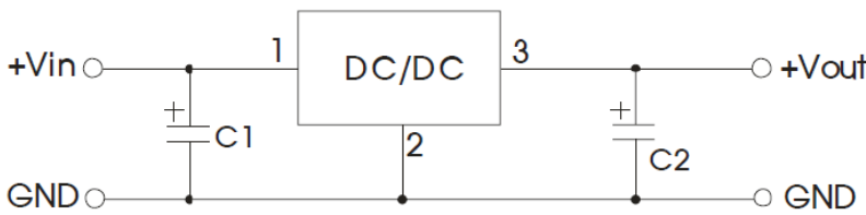
圖 2 典型應用電路
