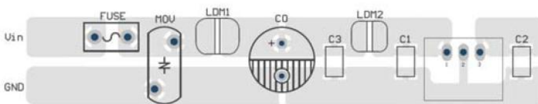
圖 5 EMC 推薦電路——PCB 布板圖
